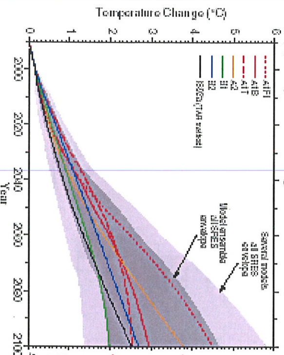
(d) Temperature change
