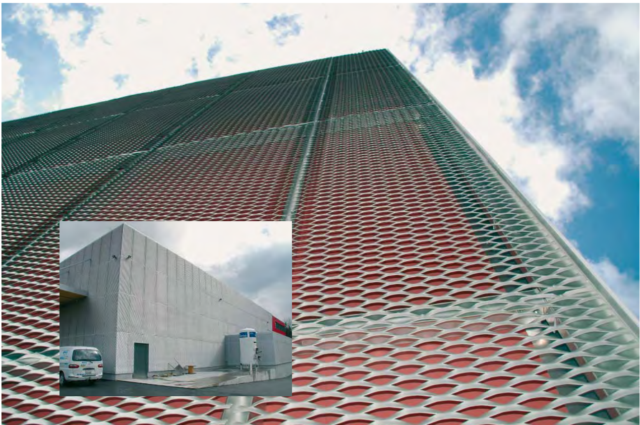
Alternative Aussenverkleidung: Diese grösstenteils mit Streckmetall eingekleidete Fassade eines Fabrikationsbetriebes ist für Vögel unbedenklich. Bei Öffnungen von maximal 2 cm Durchmesser besteht auch keine Gefahr, dass Vögel in die Fassade eindringen.
