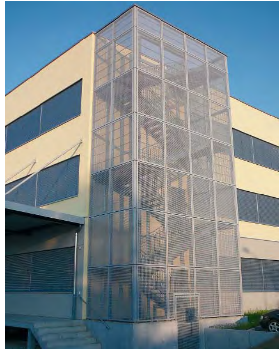
Metallgeflecht: lichtdurchlässig, wirtschaftlich, vogelfreundlich.
