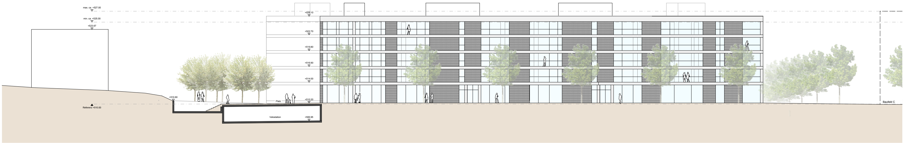
FASSADE WEST 1:400
