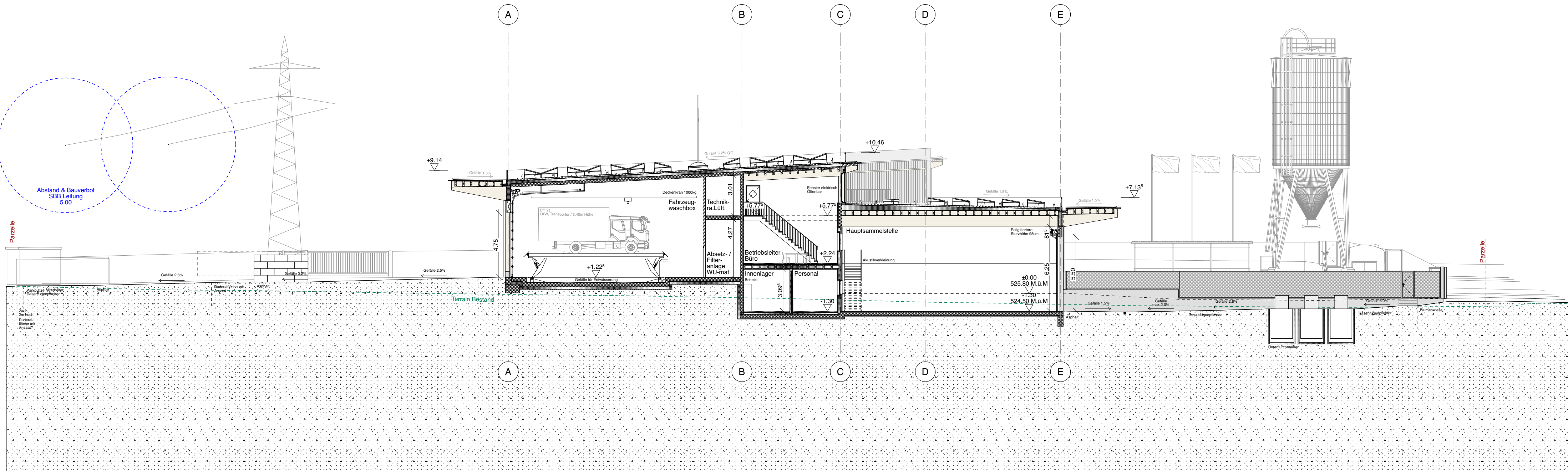
Querschnitt 19-19 (Waschbox Unterhalt - Büro Hauptsammelstelle)
