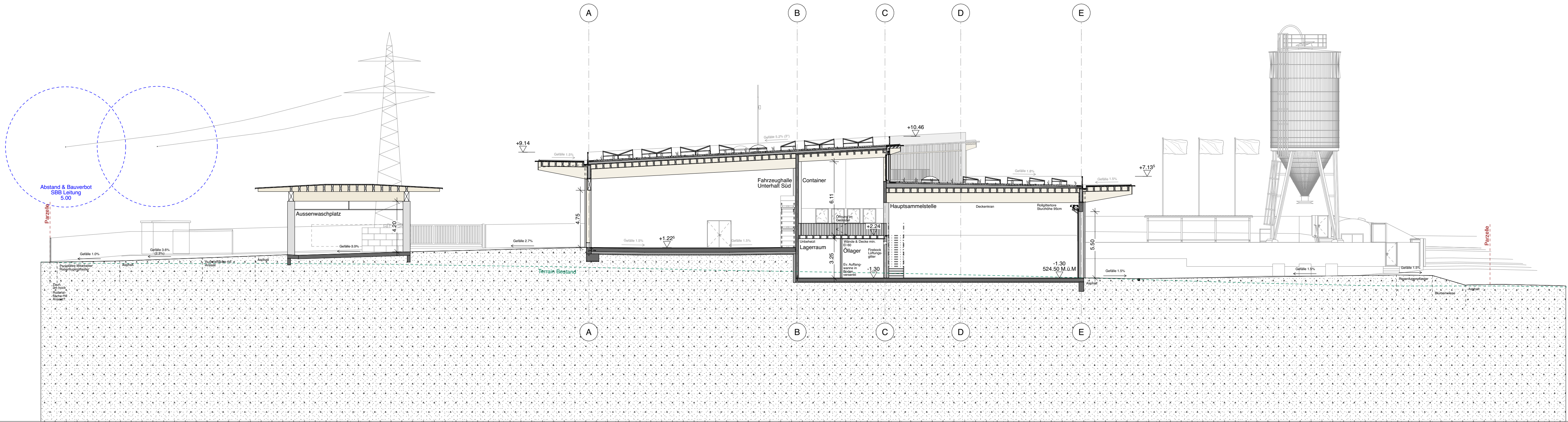
Querschnitt 24-24 (Unterhalt - Hauptsammelstelle)
